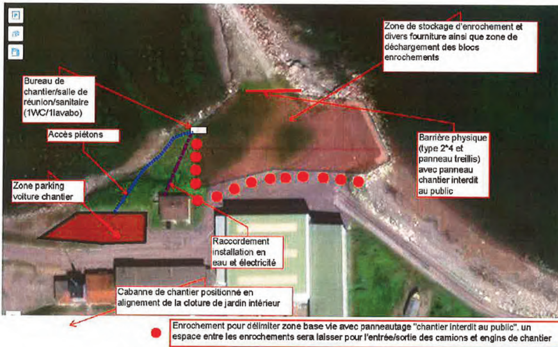
ANNEXE 1 : Plan des installations de chantier (Source : Société de Travaux Publics STP, Juillet 2019)
