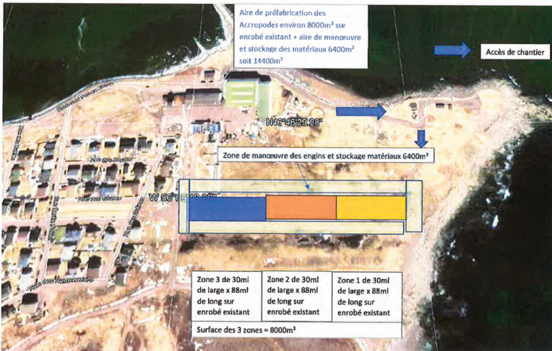
ANNEXE 2 : Plan des aires de préfabrication et stockage des accropodes (Source : Société de Travaux Publics STP, Juillet 2019)
